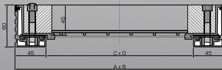
3 Joints sur deux niveaux
